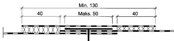
Fig. 5.4.4 Takfolie. Feste gjennom omlegg med overdekning
