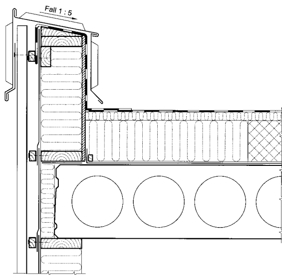
Fig 3.2.2. Lufttette overganger tak/parapet og parapet/vegg samt lufttett takkonstruksjon er viktig.
