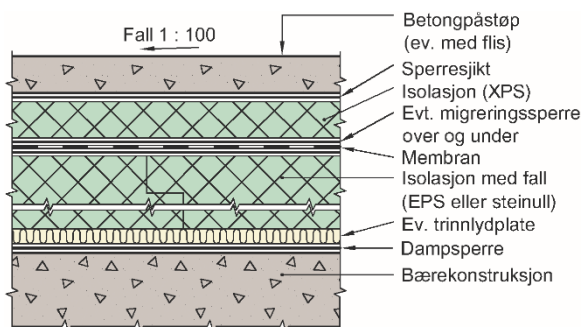
Fig 1c. Duo terrassekonstruksjon
