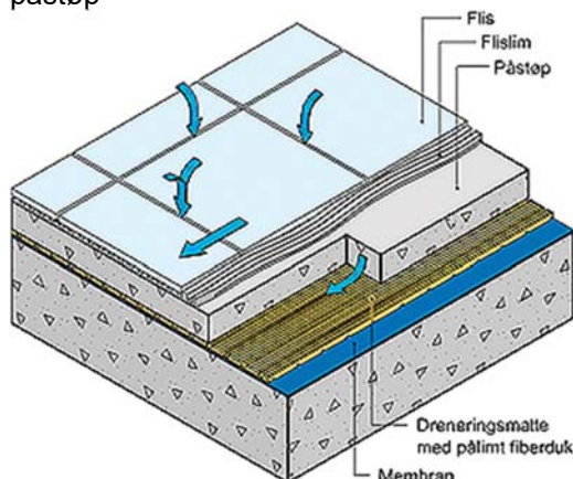
Fig. 8.7 Prinsipløsning for dreneringsmatter oppå underliggende membran Matta bidrar til å få vann transportert ut av konstruksjonen og gjør at underlag og påstøp kan bevege seg uavhengig av hverandre.
